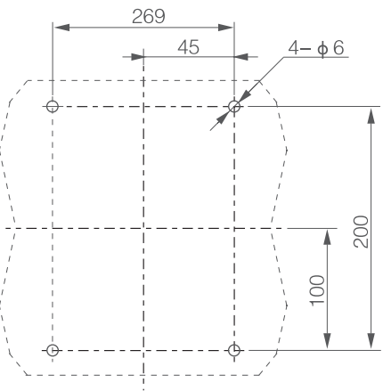
4P : Установка на монтажную панель
