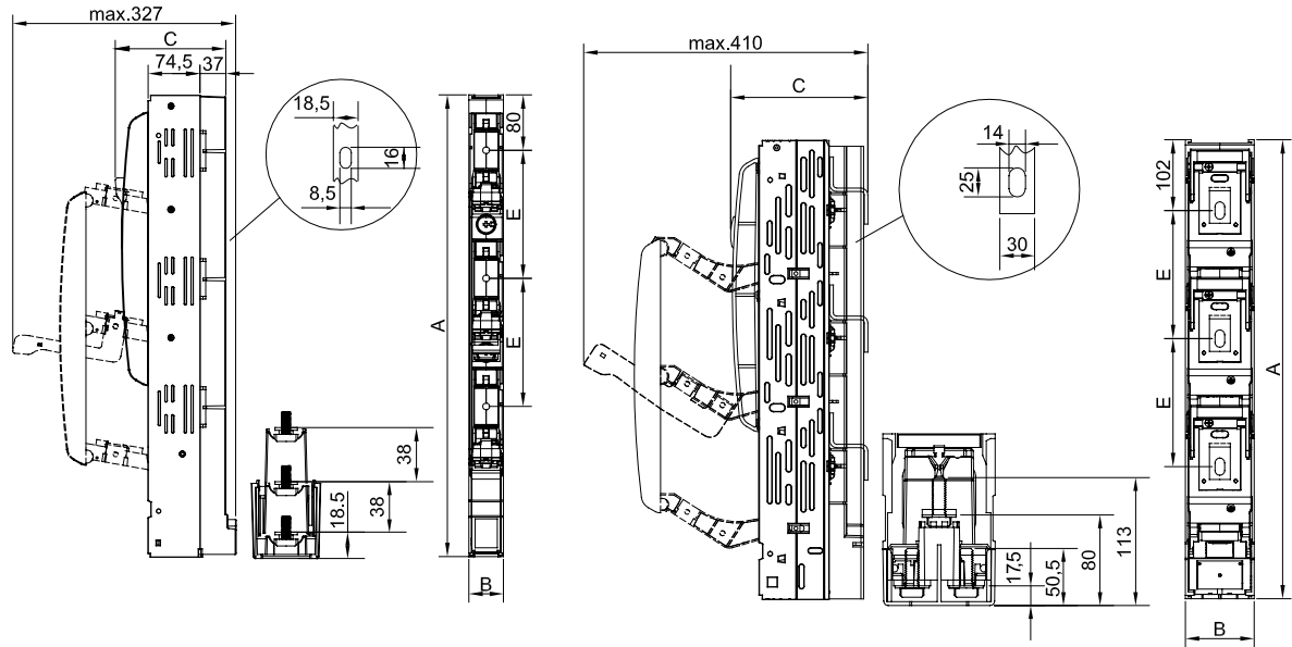
160 Габаритные и установочные размеры
