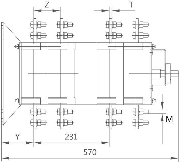
YCHGLZ1 2000-3200A с боковым управлением
