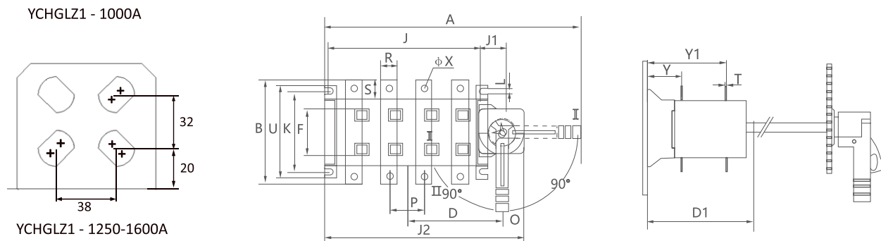
YCHGLZ1 160-1600A управление с дверцы шкафа
