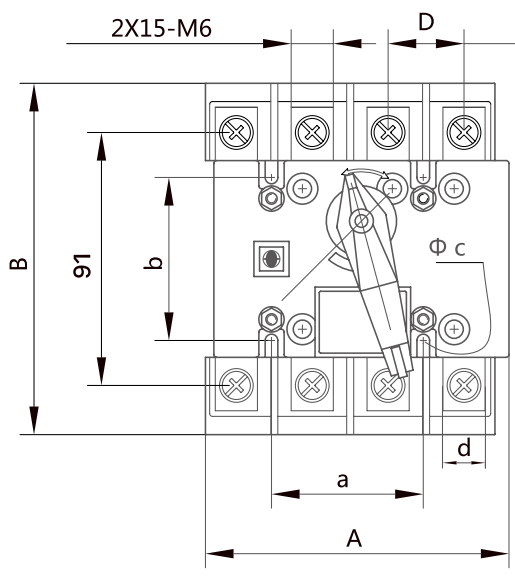
YCHGL(B) 100A прямого управления
