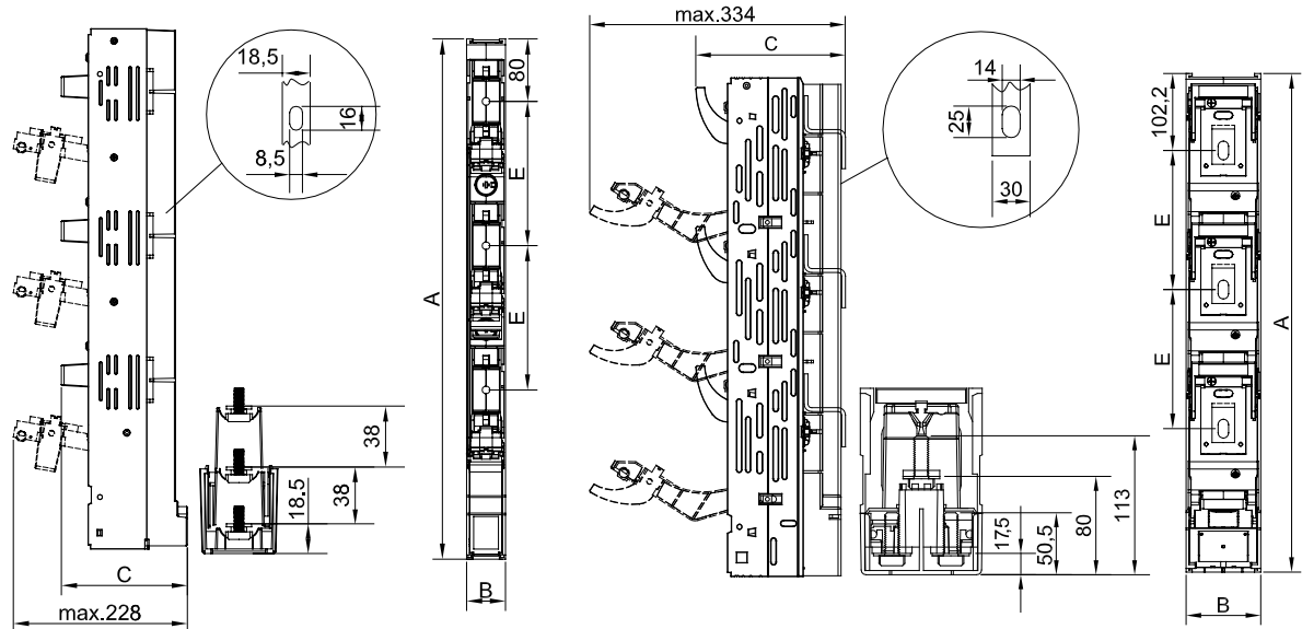
160 Габаритные и установочные размеры
