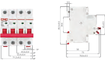
Модульный автоматический выключатель YCB9-80M максимальный ток КЗ 6кА
