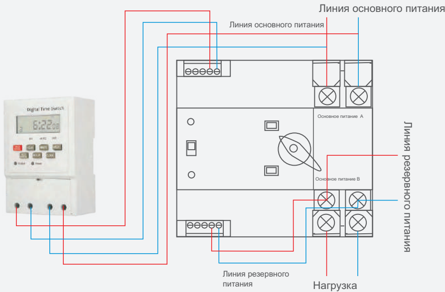
Режим переключения по времени YCQ4R Рис.5
