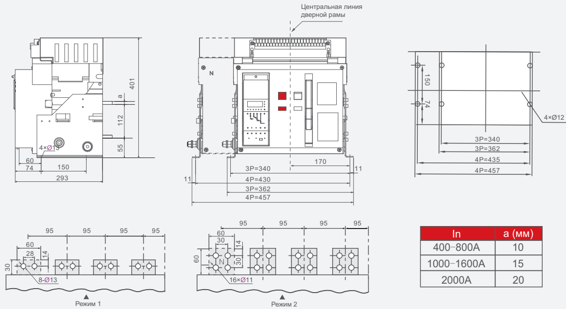
Габаритные и монтажные размеры (In равен 2000 А, 3 или 4 полюса)
